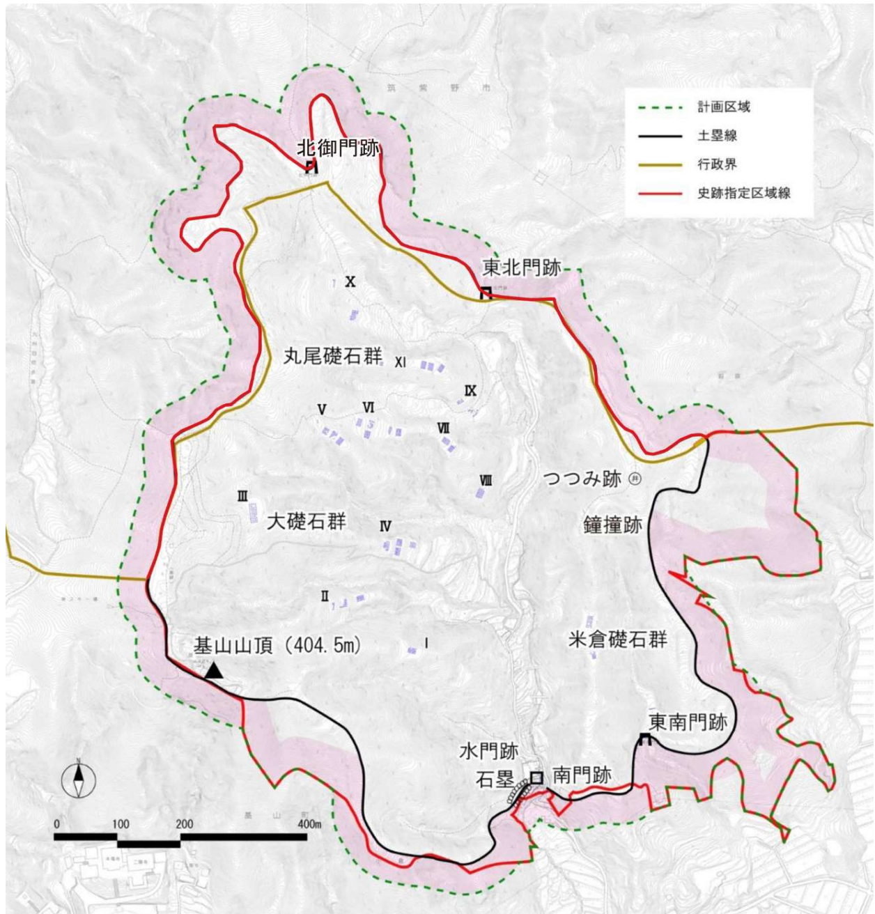
図 24. 設定区域図
