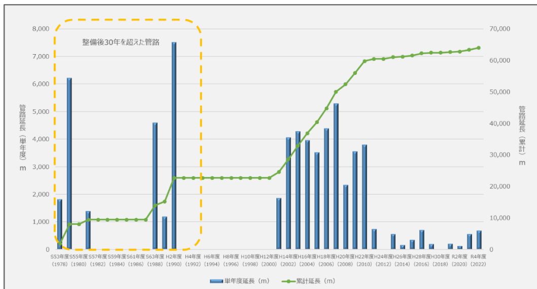
図・表 3 - 1 年度別下水道管渠布設延長 (地区全体)
