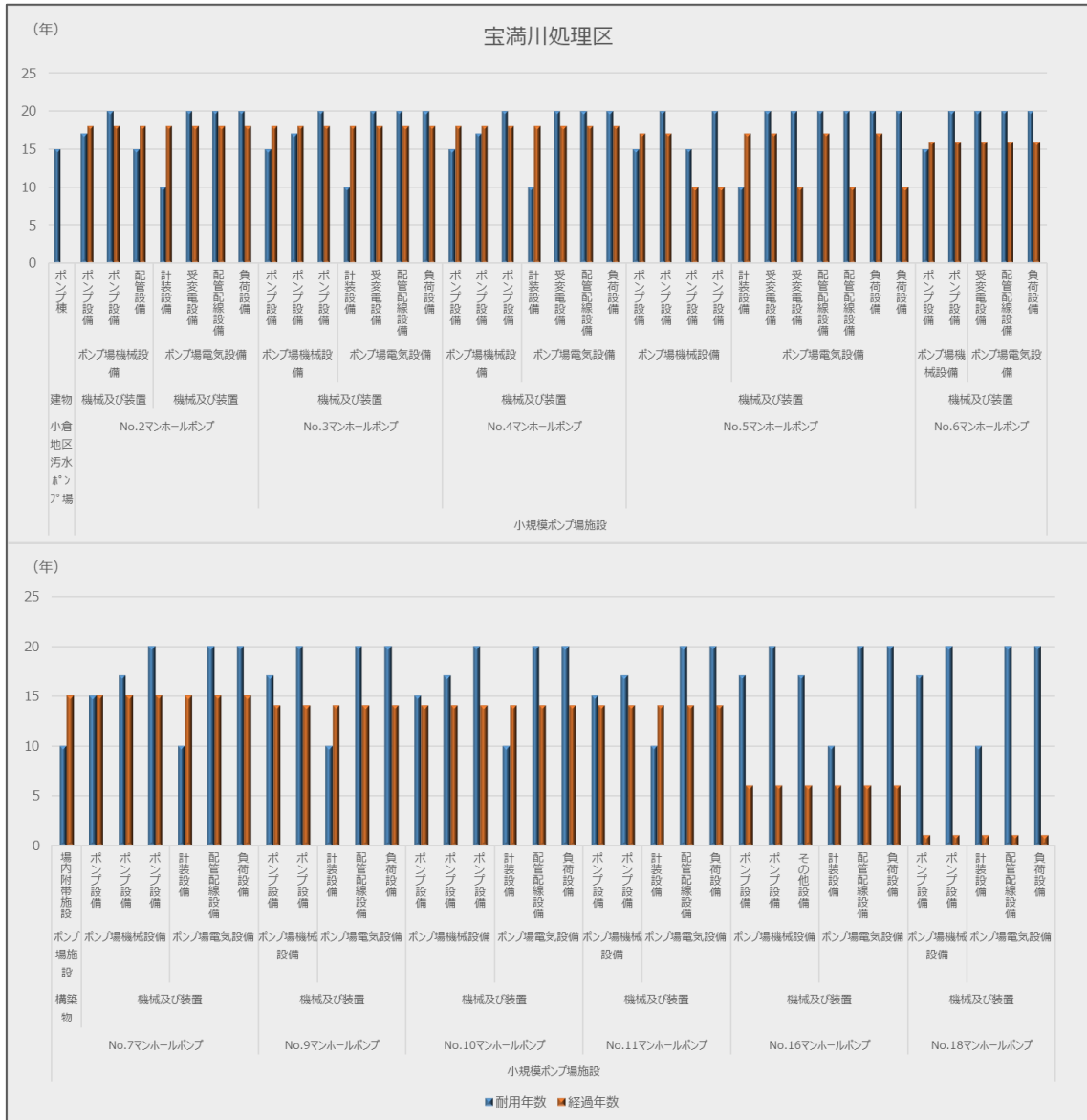
図・表 3-12 宝満川処理区 施設及び設備等の耐用年数と経過年数
