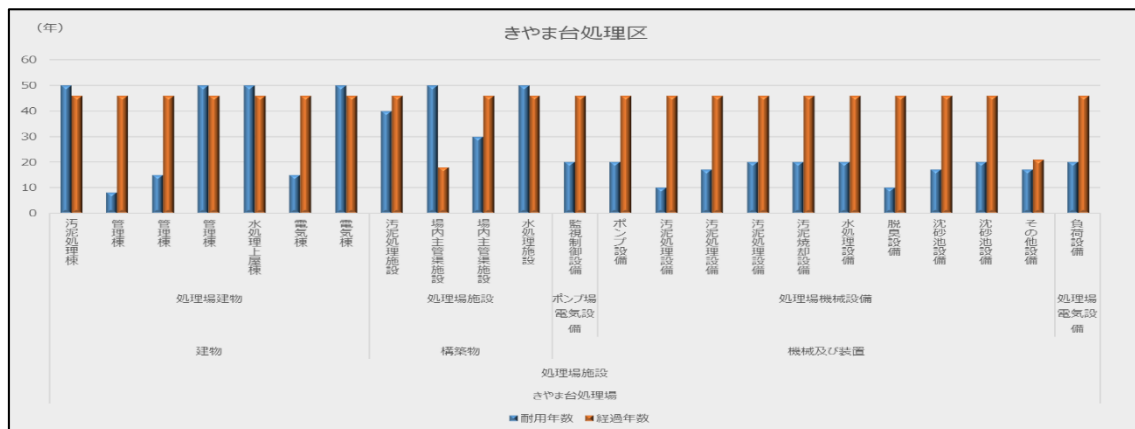
図・表 3-10 きやま台処理区 施設及び設備等の耐用年数と経過年数
