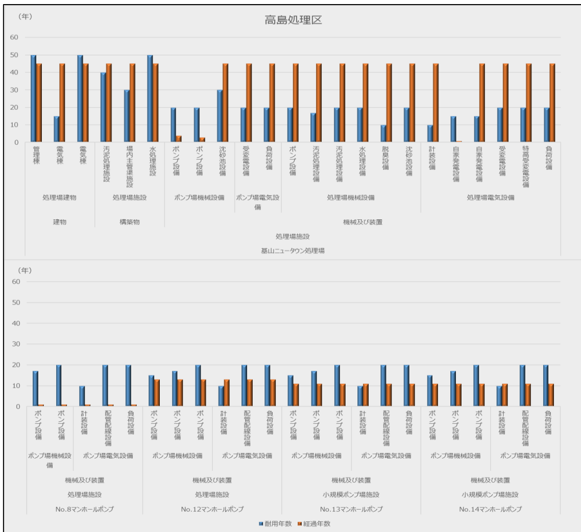
図・表 3-6 高島処理区 施設及び設備等の耐用年数と経過年数
