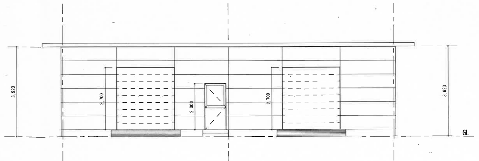
南側立面図
