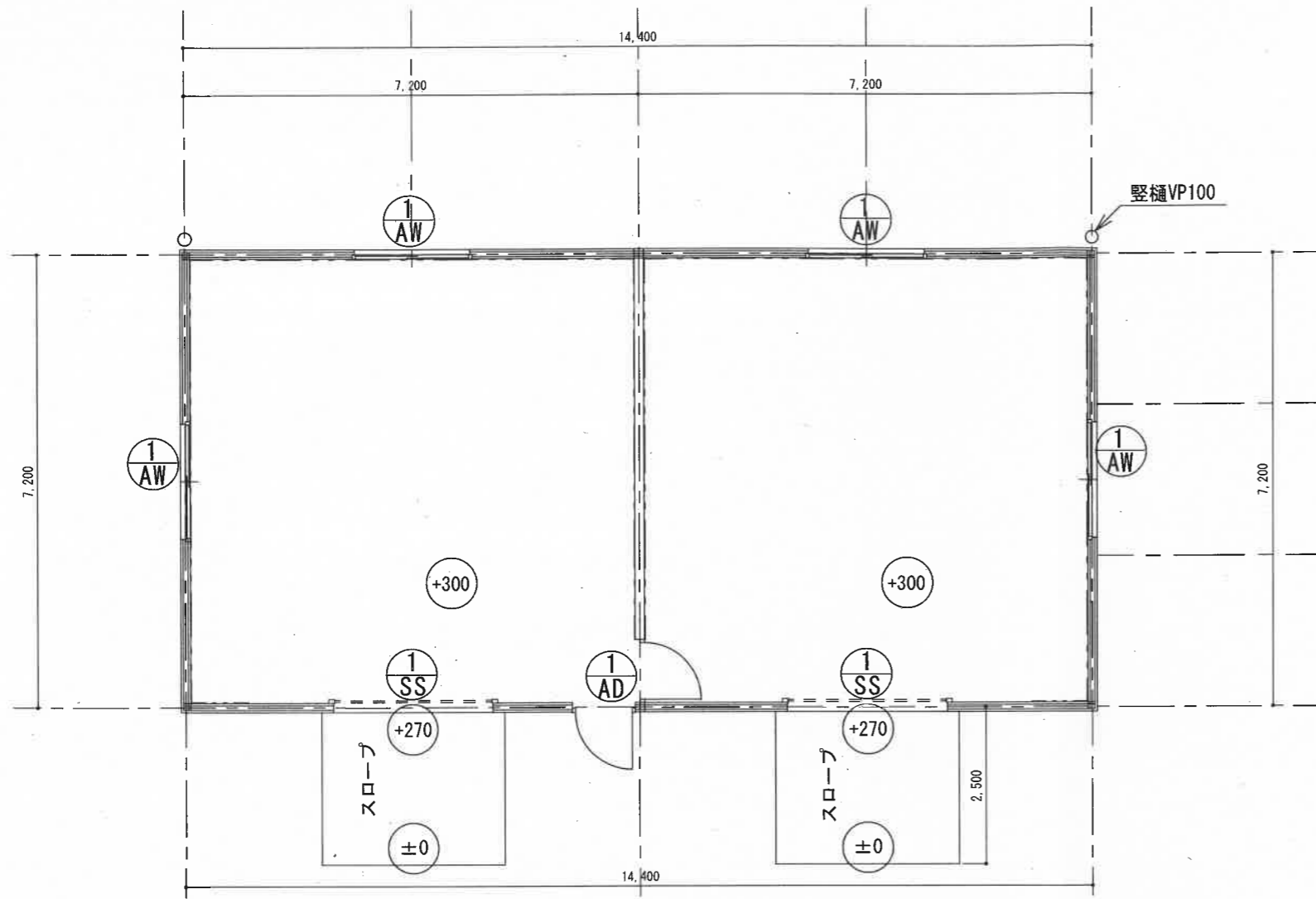
平面図
