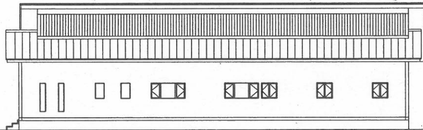
東立面図
