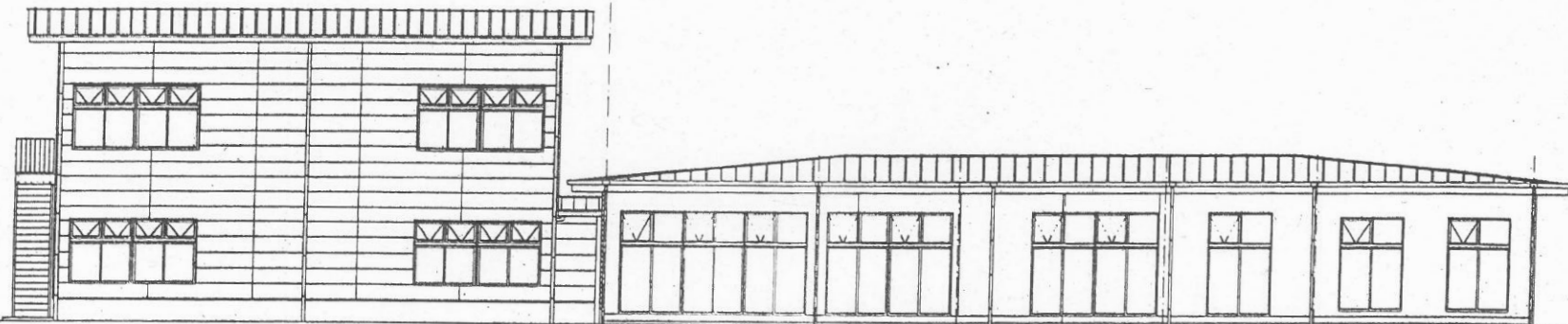
南立面図
