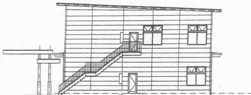
西立面図
