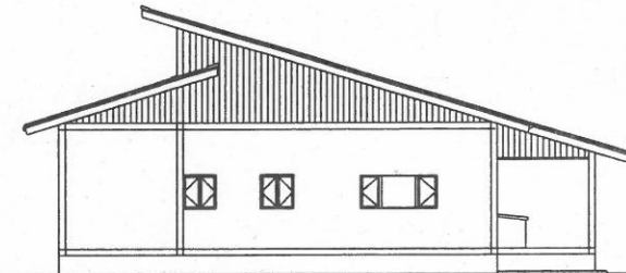
北立面図
