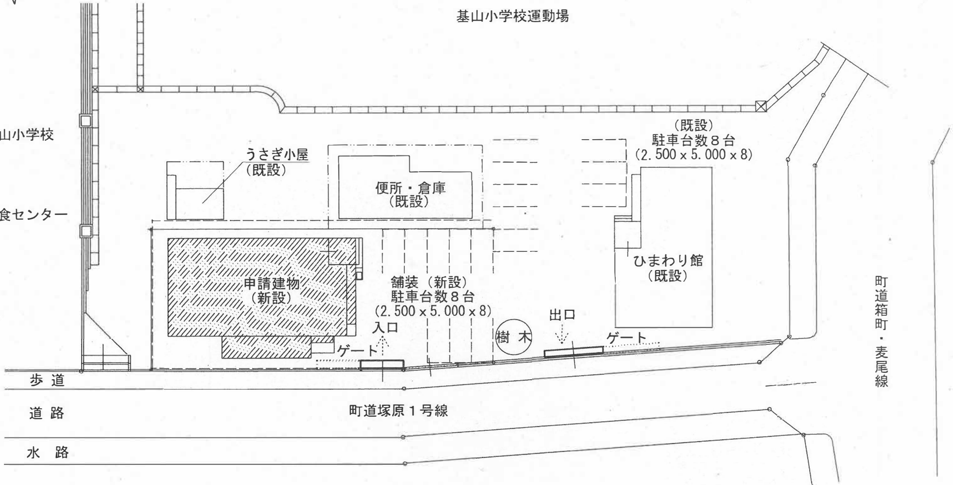
配置図
